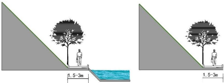
图 4—7—2 游览步道滨水及山地步道横断面图
